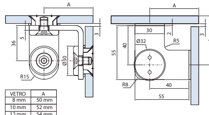
RA-011-S con tappo svasato RA-011-S with countersunk point RA-011-S mit versenkte Punkthalter
