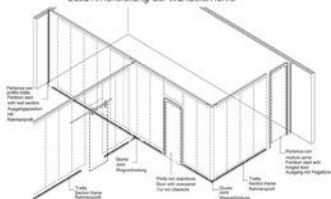
Profilo parete Partition profile Rahmenprofil
