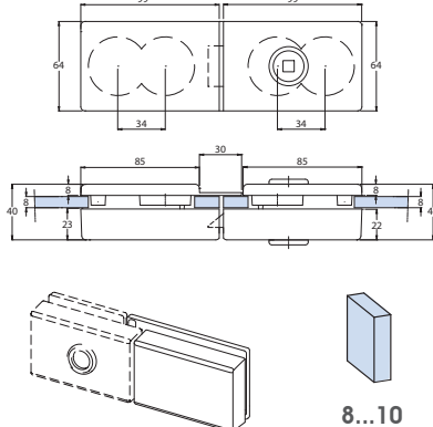
Cerniere Pag 224 Hinges Page 224
